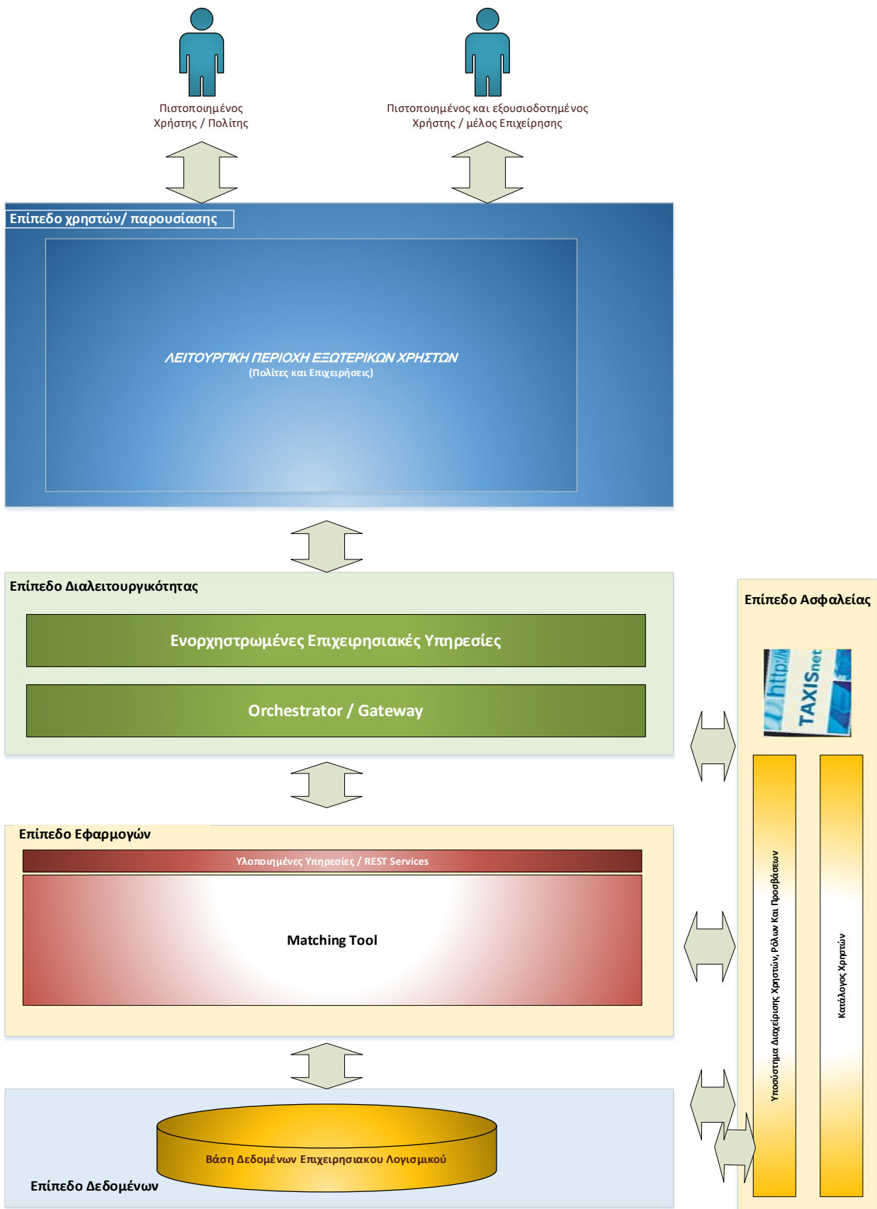
Εικόνα 1 - Λογική Αρχιτεκτονική
